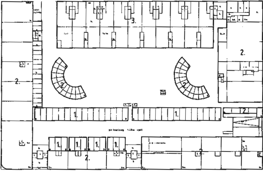
beg. grond 1:200
